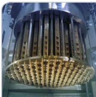
Reaktoripaineastian ylemmät sisäosat, (Chooz 1, Ranska).
