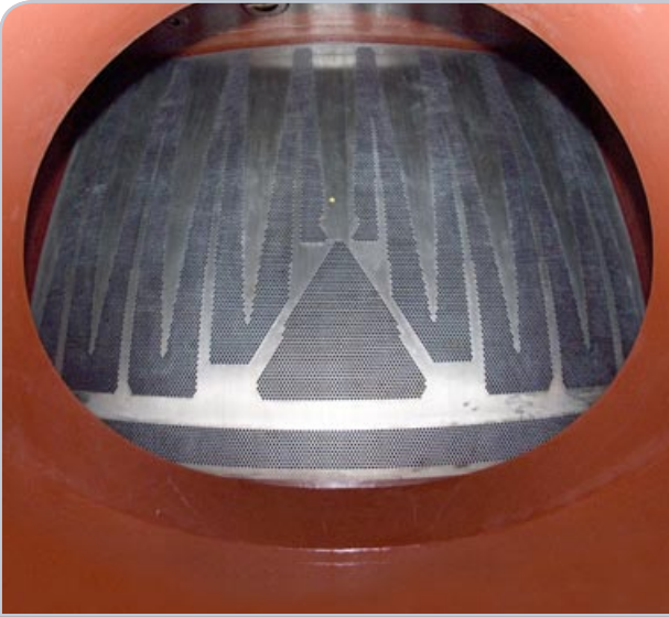
Lauhdutinlohkosten jäähdytysvesituubien konstruktio (lauhduttimen tuubilevy).
